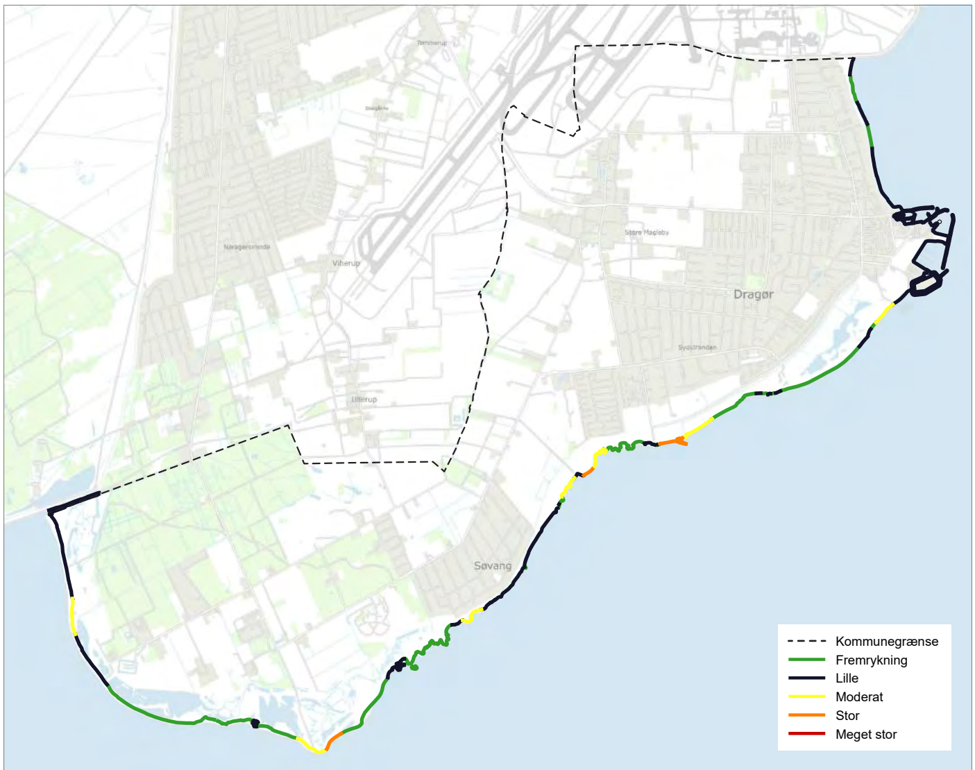
Figur 1 Retningslinjekort. Kortet viser, hvilke strækninger, der udsættes for kronisk erosion. Kyster med moderate til store erosionsrater holdes under observation.
