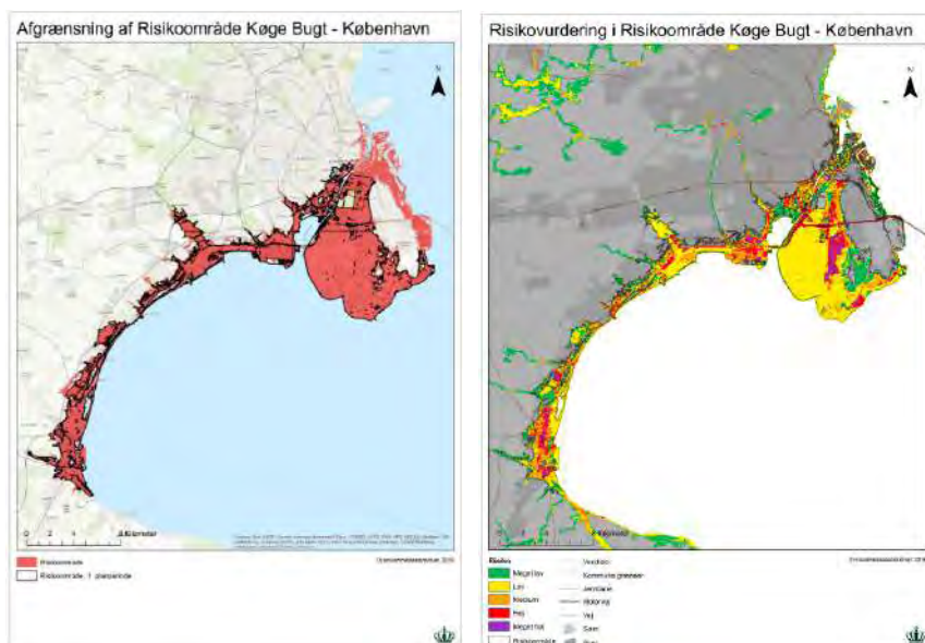
Figur 3 Fra Kystdirektoratet – Oversvømmelsesdirektivet 2018, Hovedrapport. Revurdering og ajourføring af risikoområder for oversvømmelse fra hav og vandløb.
